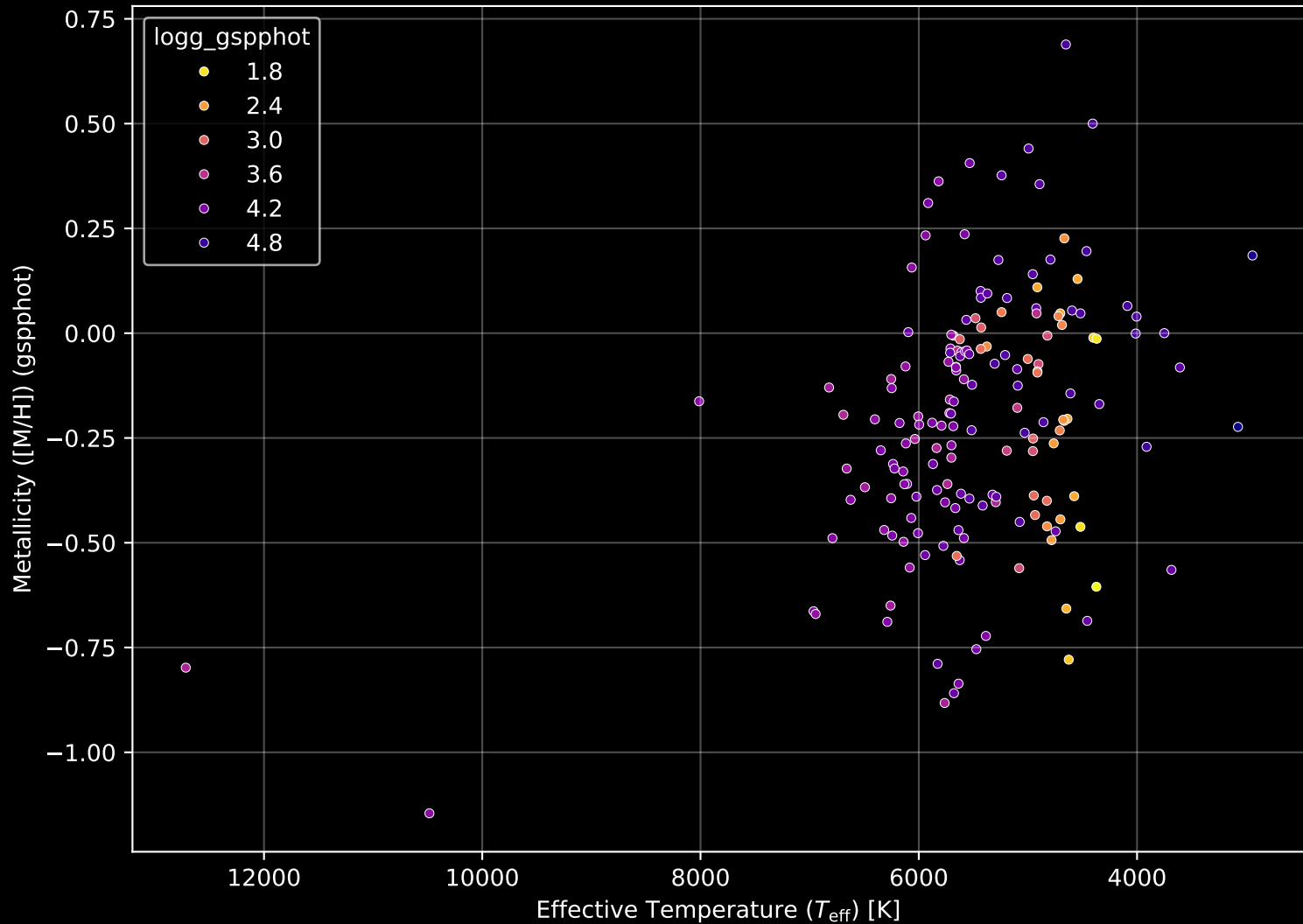
APOGEE DR17 Field: [271-32-O_TESS] Stellar Population Parameters (n= 171)
